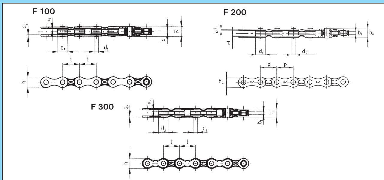
Valčkové reťaze jednoradové podľa normy ČZ.
