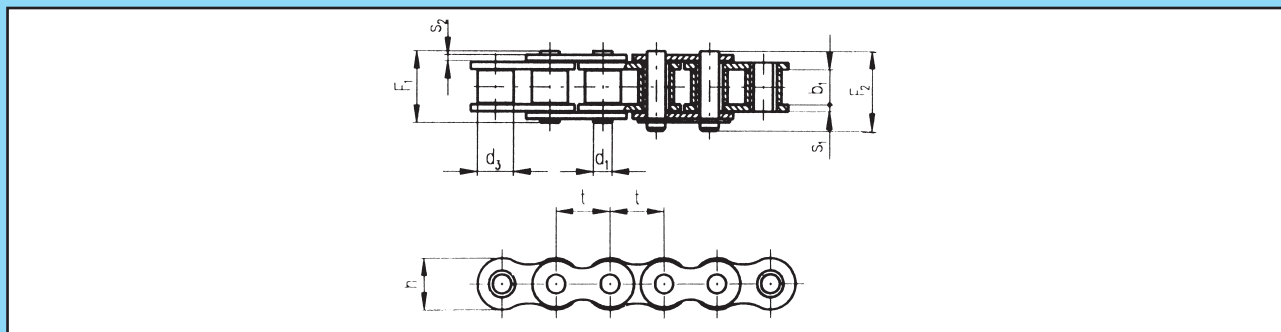
Valčkové reťaze jednoradové podľa normy ČZ.
